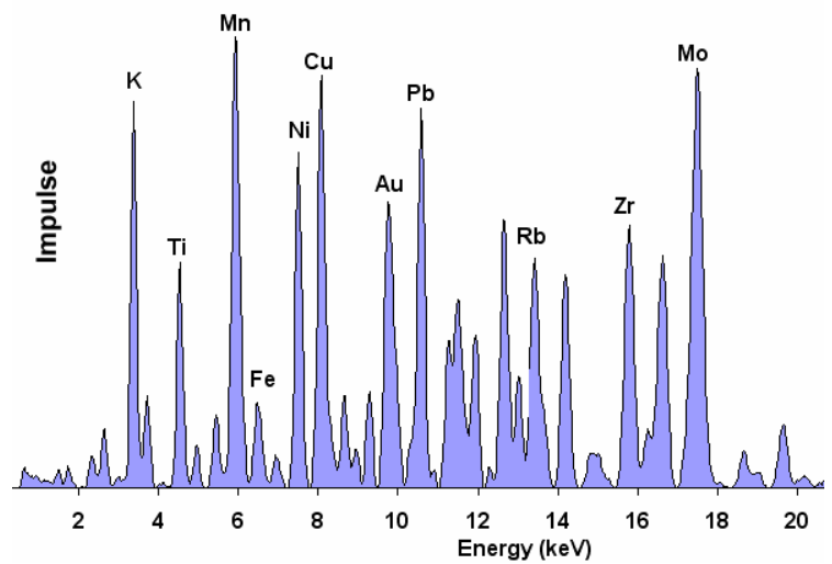
Ein XRF-Spektrum (jedes Element hat andere Energien, die Konzentration liefert die Anzahl Impulse)
